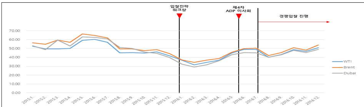
[그림] 2015 ~ 2016년도 국제유가(WTI, Brent 및 Dubai) 현황
